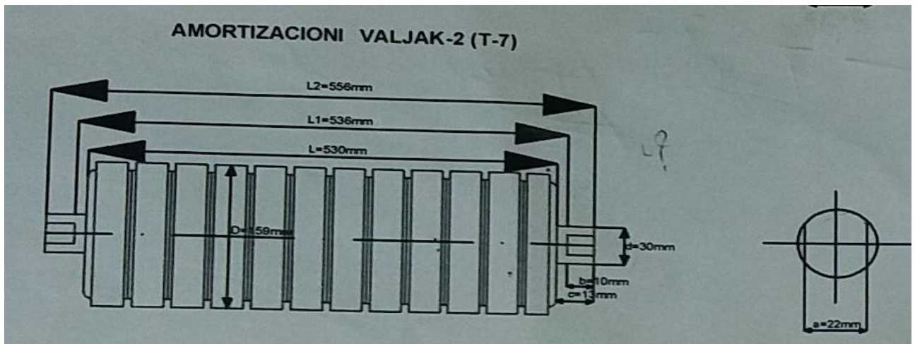
4. Slika 4: Amortizacioni valjak 159x30x530mm a=22mm
