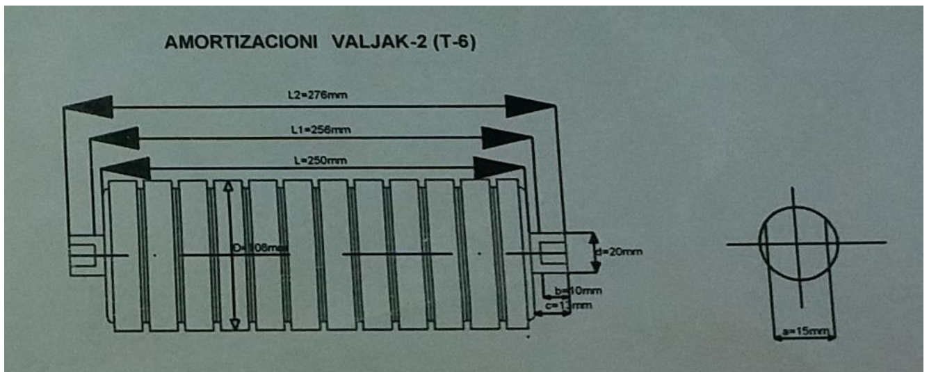
3. Slika 3: Amortizacioni valjak 108x20x250 mm a=15mm
