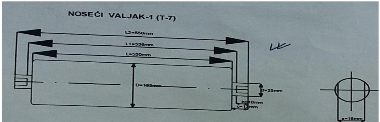
2. Slika 2: Metalni noseći valjak 133x25x530 mm a=18mm
