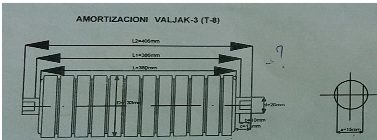
5. Slika 5: Amortizacioni valjak 133x20x380mm a=15mm
